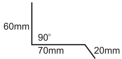
Apron Flashing
