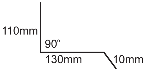
Apron Flashing
